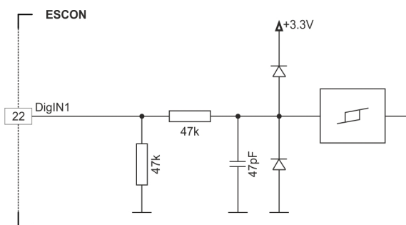
Figura 3-5 Circuito de DigIN1
