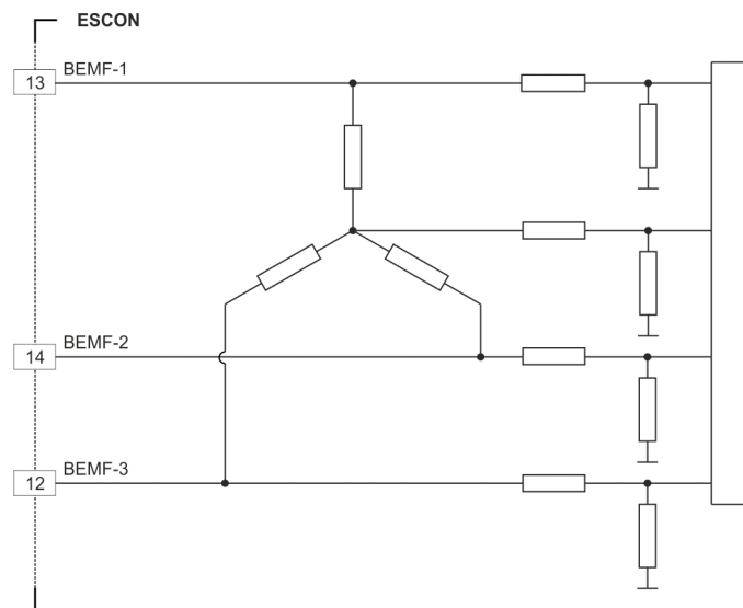
Figura 3-4 Conexión de señales de FCEM
