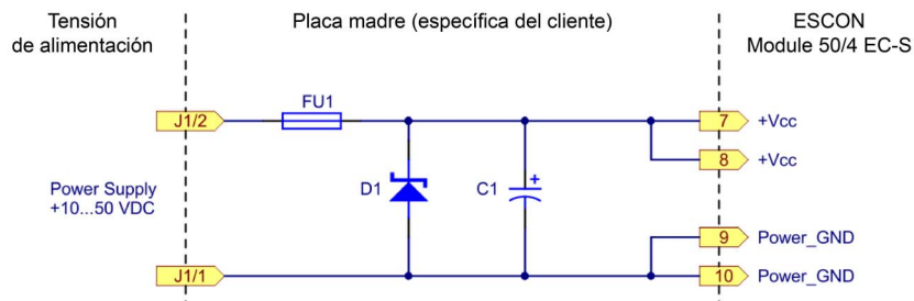
Figura 5-17 Conexión del cable de alimentación
