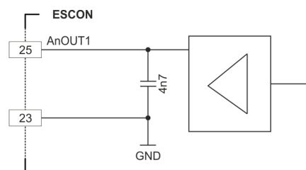
Figura 3-11 Circuito de AnOUT1 (similar también para AnOUT2)
