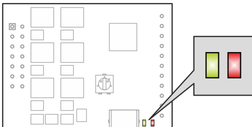
Figura 3-14 LEDs – Lugar de montaje
